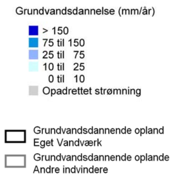
Figur 4.2 Grundvandsdannelse til kalkmagasinet i mm pr. år og grundvandsdannende opland til Magleby Vandværk.
