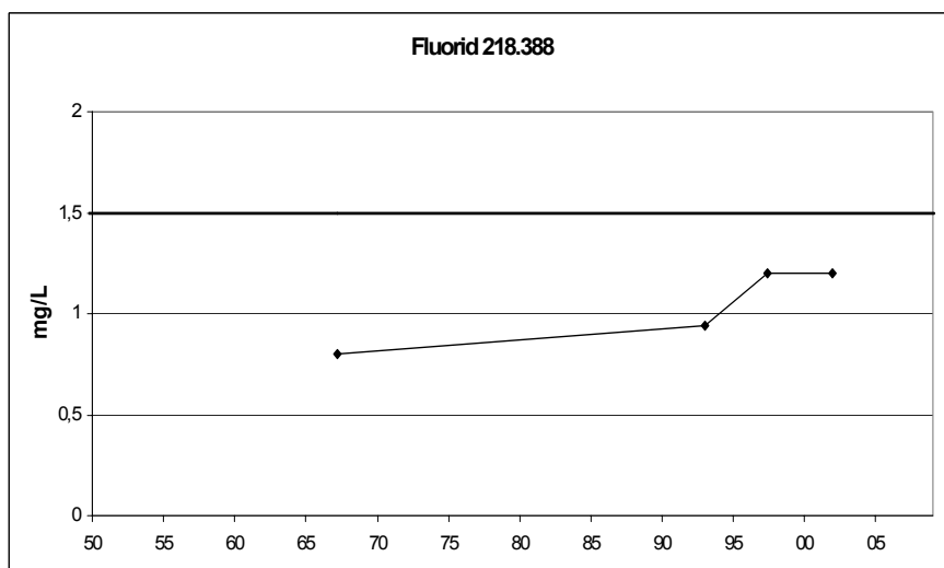
Figur 3.4. Udviklingen i fluorid i råvand, boring 218.388. Grænseværdien for rentvand er markeret med en fed linje.
