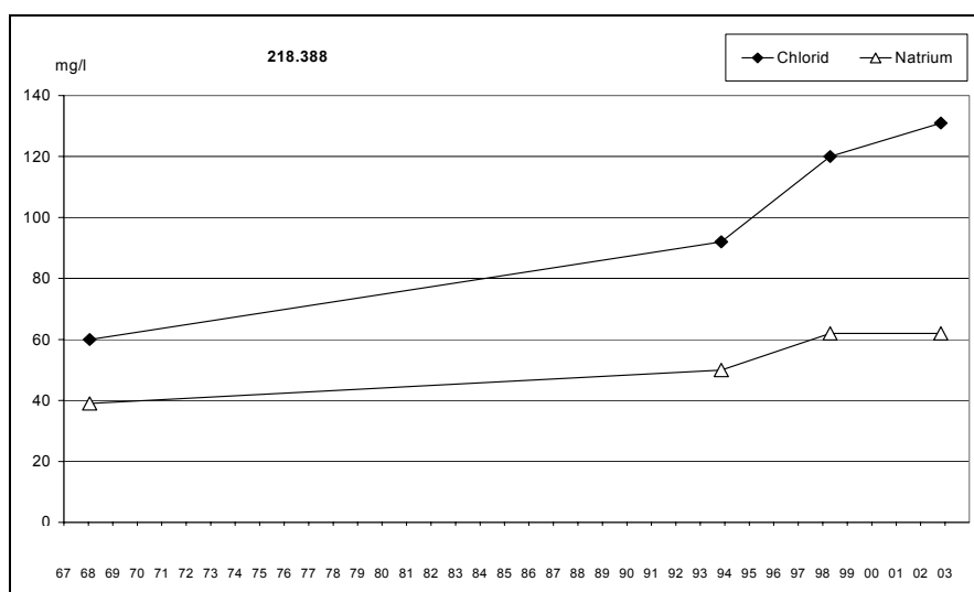
Figur 3.3 Udviklingen i chlorid og natrium i råvand, boring 218.388 i perioden 1967-2003.
