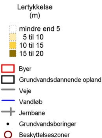
Figur 4.1 Lertykkelse over det primære grundvandsmagasin.
