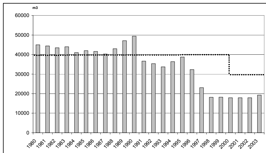
Figur 3.2 Indvundne årlige vandmængder i perioden 1980-2003. Den stiplede linie angiver indvindingstilladelsens størrelse.
